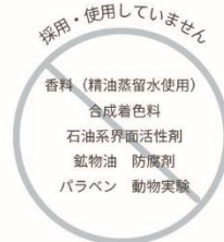
黒文字 - kuromoji -
